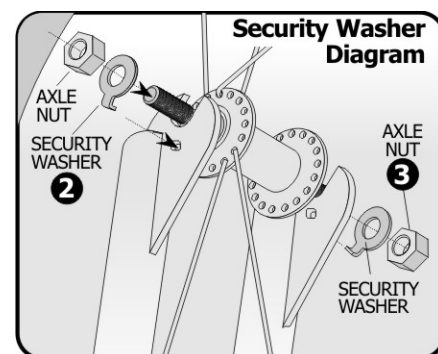
Vyobrazení bezpečnostní podložky
