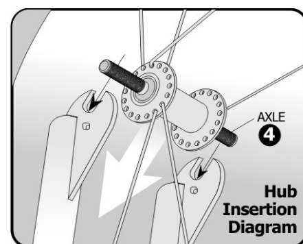
4 - Osa Náboj vyobrazení montáže
